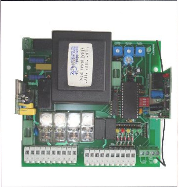
Fig. 2 - SS-PM8 - RICEVENTE RADIO A SCHEDA - WITH RADIO RECEIVER CARD - AVEC RECEPTEUR A FICHE
