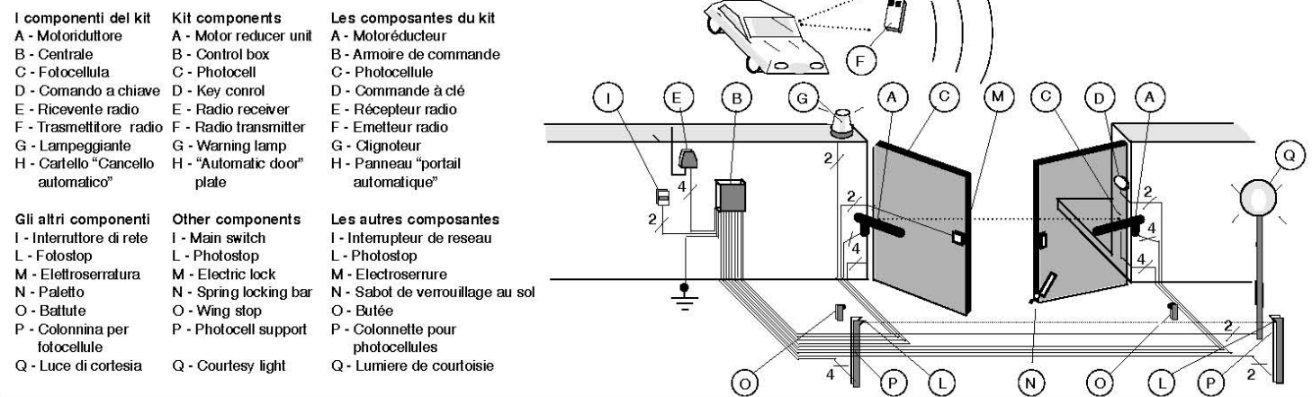
Fig. 16 - SS-PM8 CARATTERISTICHE TECNICHE - TECHNICAL DETAILS - DONNÉES TECHNIQUES
