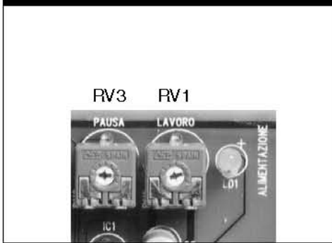
Fig. 8 - REGOLATORE DI COPPIA - TORQUE ADJUSTMENT CARD - REGULATEUR DE COUPLE
