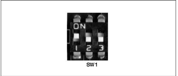
Fig. 9 - DIP DI SELEZIONE PROGRAMMA - PROGRAM SELECTION DIP - DIP DE SELECTION PROGRAMME
