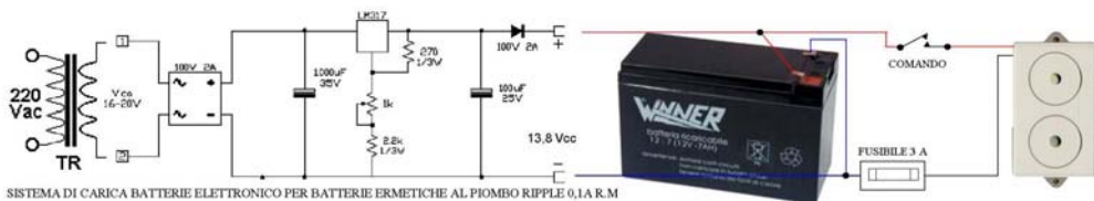
SISTEMA DI CARICA BATTERIE ELETTRONICO PER BATTERIE ERMETICHE AL PIOMBO RIPPLE 0.1A R.M
