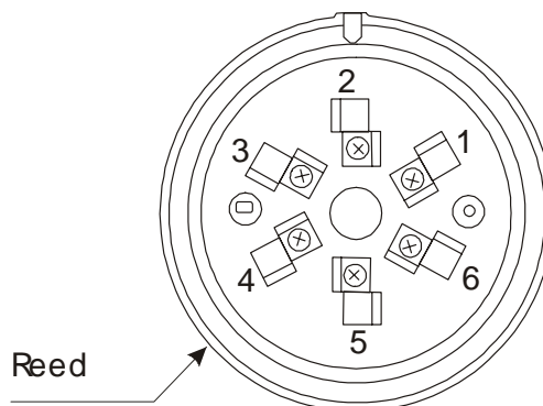
DESCRIZIONE DEI MORSETTI DELLA BASE
