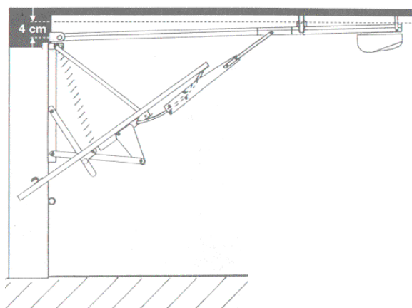
Porta basculante a contrappeso con ARC
