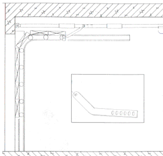
Porta basculante a contrappeso con ARC
