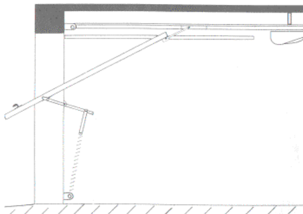
Porta basculante a molla
