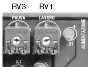
Fig. 8 - REGOLATORE DI COPPIA - TORQUE ADJUSTMENT CARD - REGULATEUR DE COUPLE
