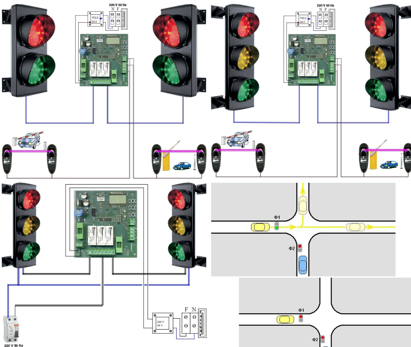
IMPIANTO SEMAFORICO 3 LUCI FUNZIONE AUTOMATICA
