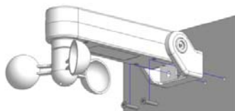
INSTALLAZIONE VERTICALE
